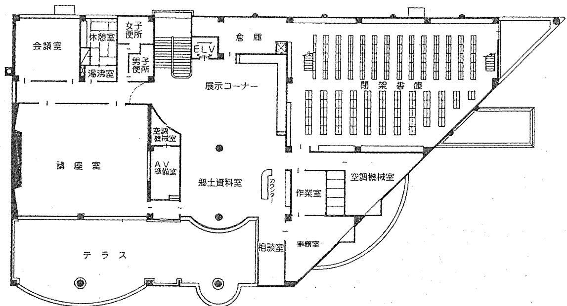
2階平面図
